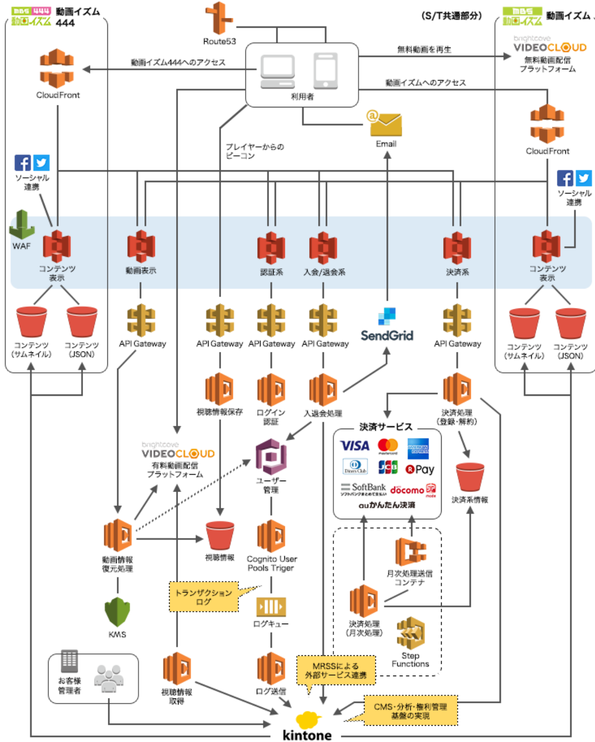
『MBS 動画イズム』動画配信プラットフォームのシステム構成図
