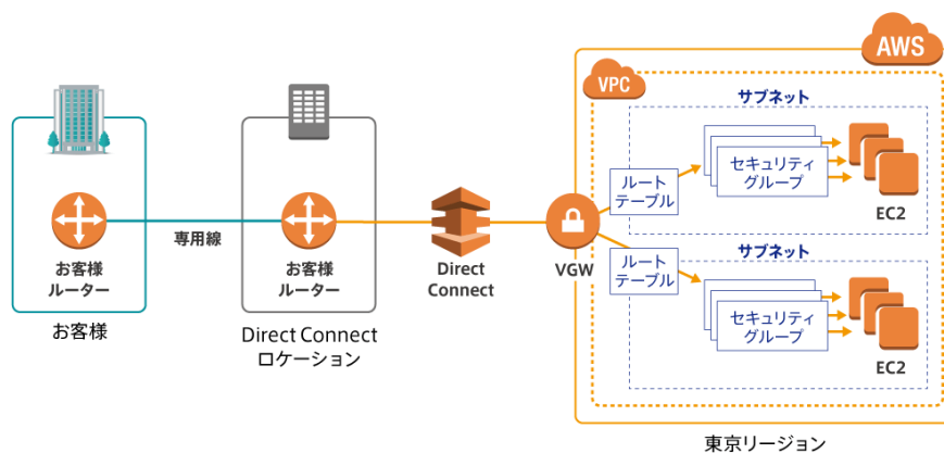
AWS Direct Connect の構成要素（ホワイトペーパーの第 5 章より）
