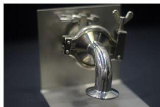
さまざまな形のスイベルジョイント製品がございますので、柔軟に配管設計が可能です。
