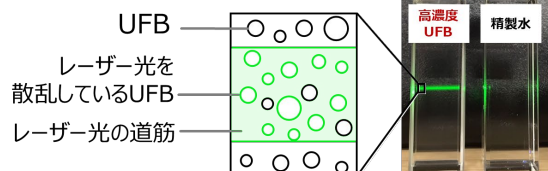
図2.レーザー光によりUFBの存在を可視化した様子
