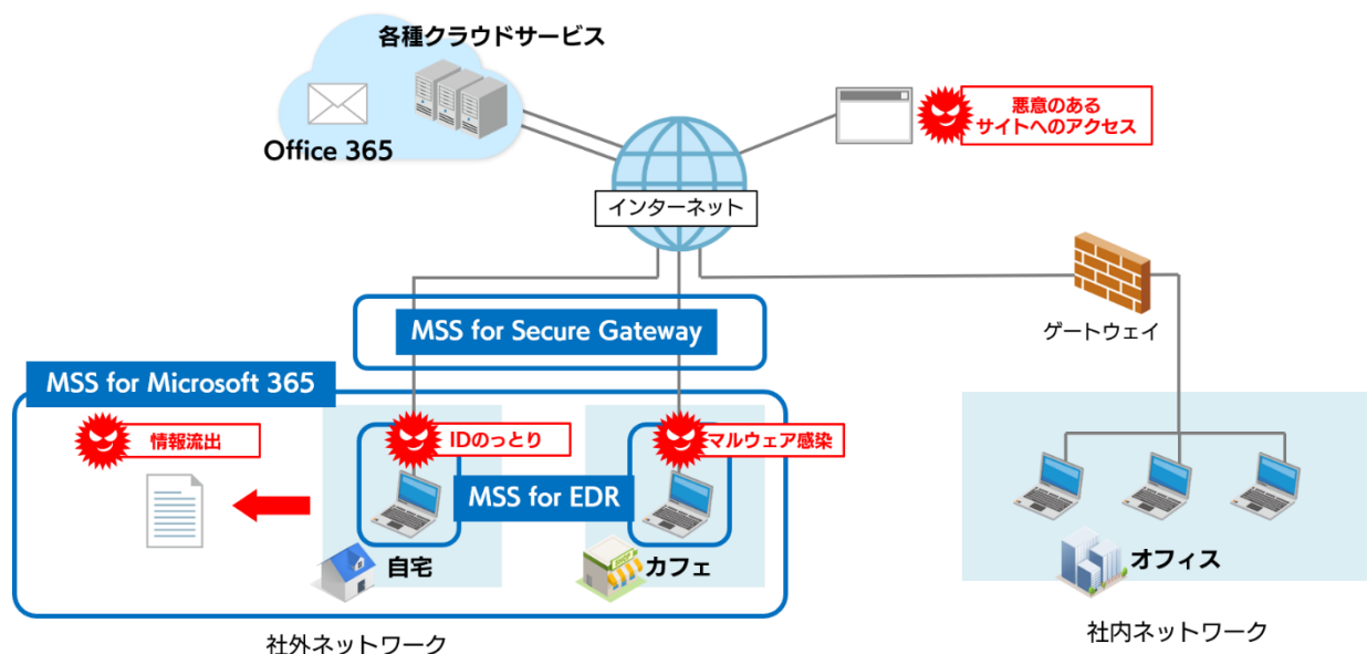
社外ネットワークにおけるセキュリティ脅威に対応するMSSのラインナップ
