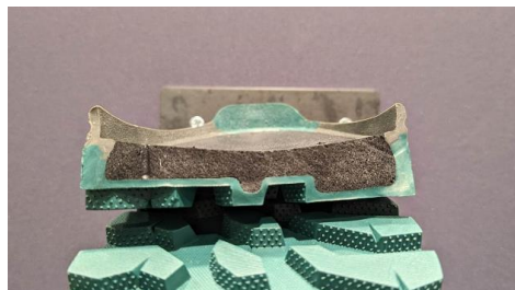
ミッドソールコア (充填PU)
