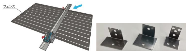
(左) 切断治具、(右) ケガキ治具
