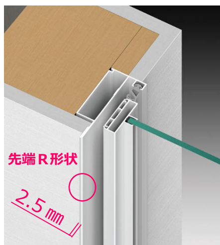
枠断面
