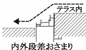
新設土間の場合の納まり
