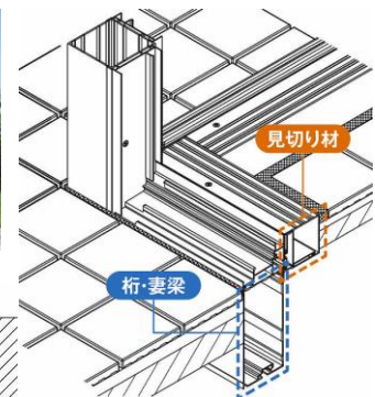
新設土間の場合の納まり
