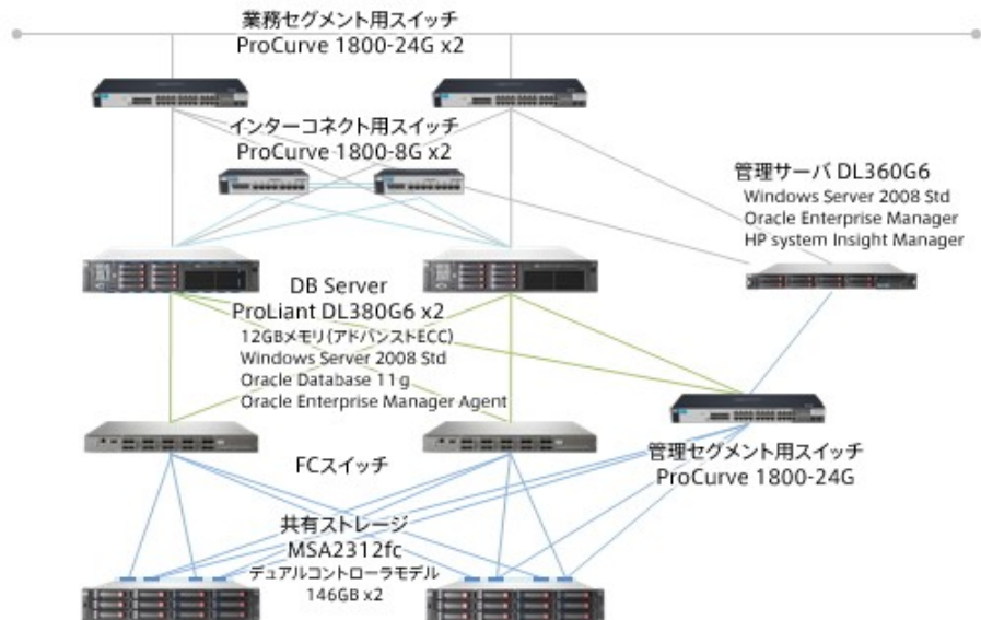
「DODAI-h ストレージ・コスト削減モデル Windows 版」システム構成図
