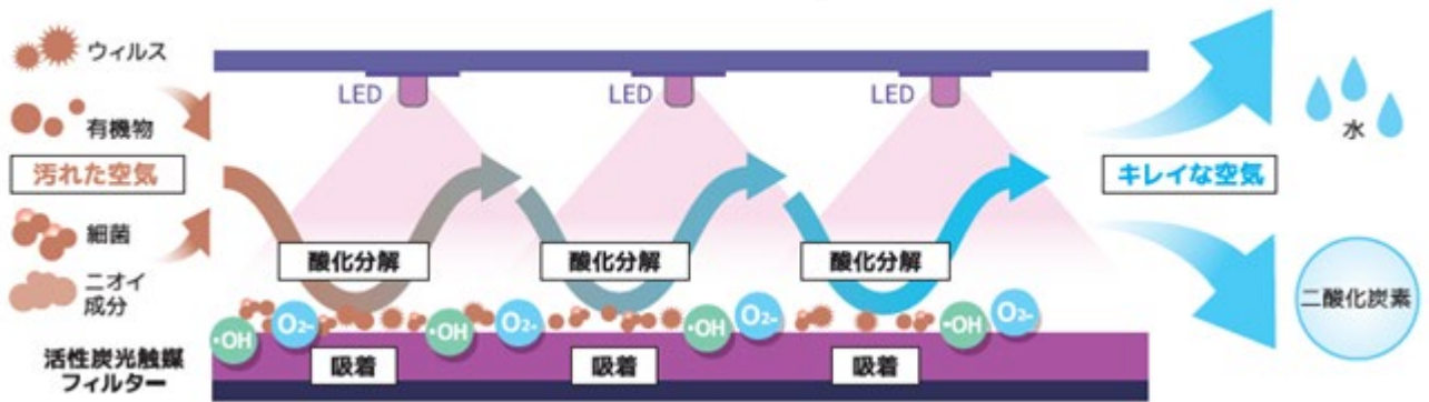
コルゲート活性炭光触媒フィルター（断面図）
