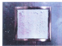
写真-2 試験体A 試験後
