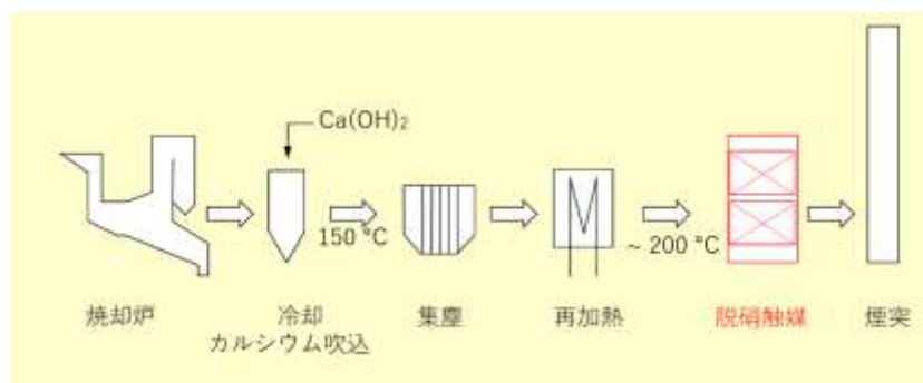
図1 ごみ焼却施設排ガス処理プロセスの例
