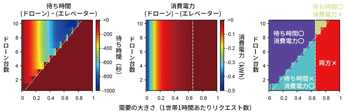
図2：エレベーターと比較した際のドローン配送の有効性
