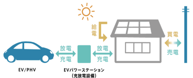
【V2H の概念図】
