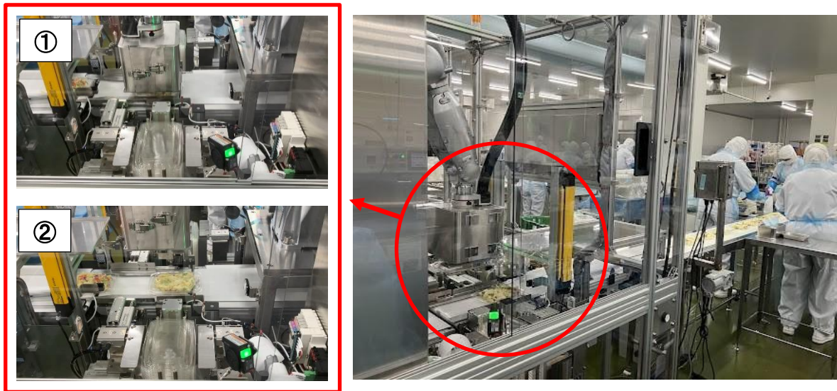
「惣菜用ふた閉めロボット」実運用の様子 写真①：手前に積み上げた容器のふたをロボットアームが取り、惣菜の容器に押し付ける 写真②：ロボットアームが上がり、ふた閉め完了
