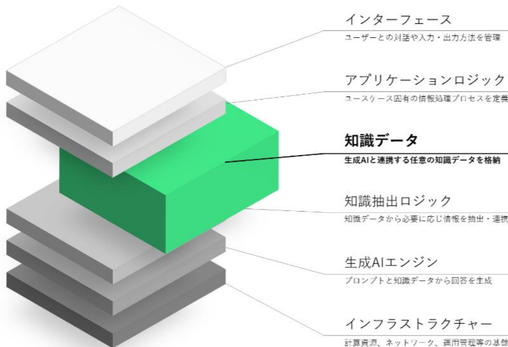
生成AIプロトタイピング環境の構造
