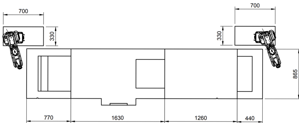
ロボットシステム平面図
