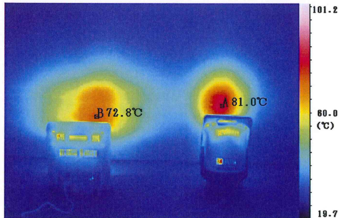
K社ハロゲンヒーター-800W エコロミ-400W (財)千葉県産業振興センター 東葛テクノプラザにて、自社調べ
