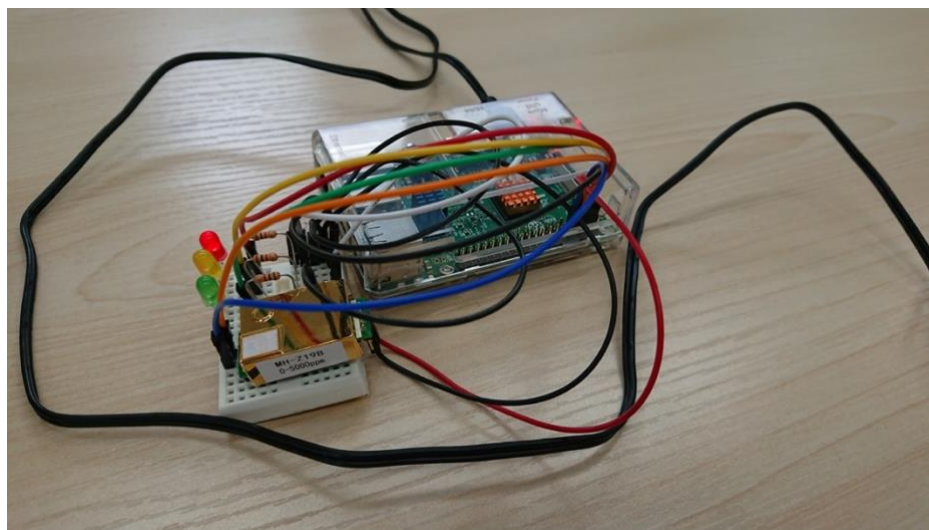
シニアジョブが自社開発し、換気による新型コロナウイルス感染防止に活用している CO2 濃度計の試作機
