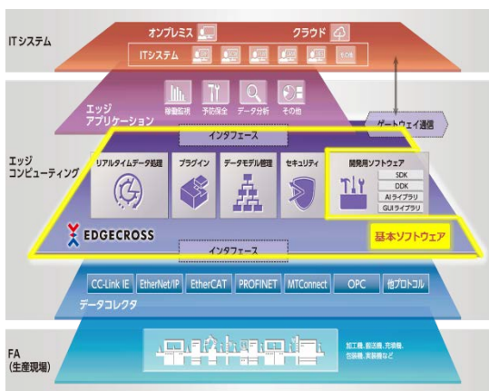
Edgecross 全体像と基本ソフトウェアの位置づけ
