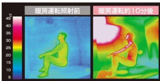
「浴室換気乾燥暖房機」温度変化 室温：10℃ 浴室面積：1坪 照射時間：10分 (メーカー調べ)
