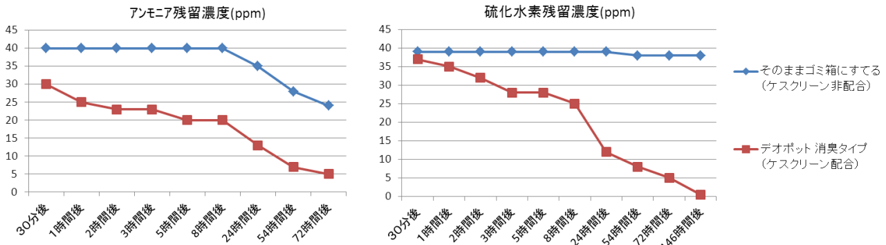
(財)化学物質評価研究機構 CERIにて、製品試験結果
