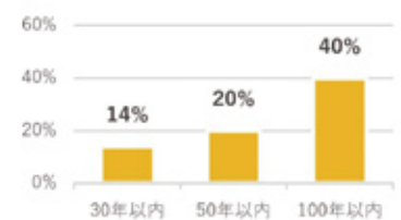
M8程度の地震の発生確率
