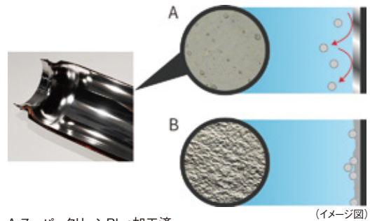
A: スーパークリーンPlus加工済 (表面がなめらかで、汚れやおいがつきにくい) B: スーパークリーンPlus未加工 (表面に小さな凹凸があり、汚れやおいがつきやすい)
