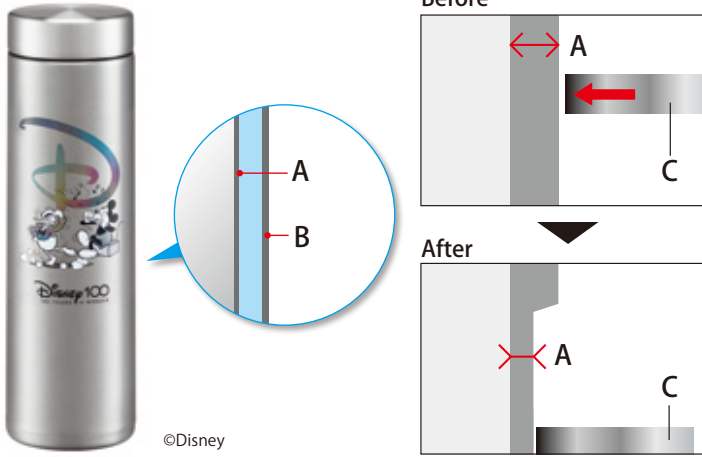
■ 真空 A:内筒の厚さ 約0.08mm B:外筒の厚さ 約0.3mm C:ローラーを押し当てる
