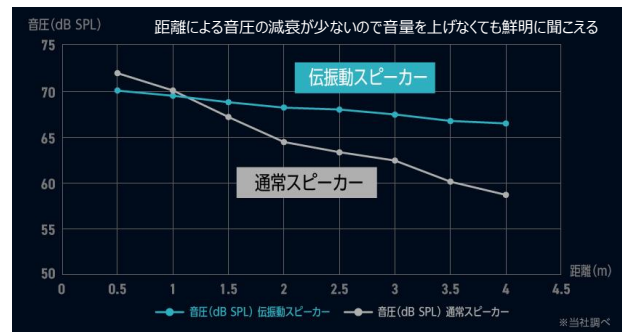
<通常のスピーカーと伝振動スピーカーの距離による音圧の比較>
