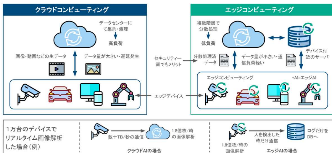
クラウドコンピューティングとエッジコンピューティングの違い (Idein作成)
