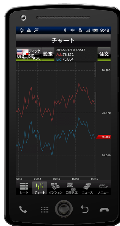
ティックチャート (Bid・Ask 同時表示)
