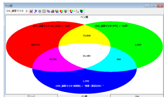
▲ベン図機能
