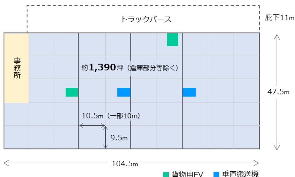
【配置図（1 階）】
