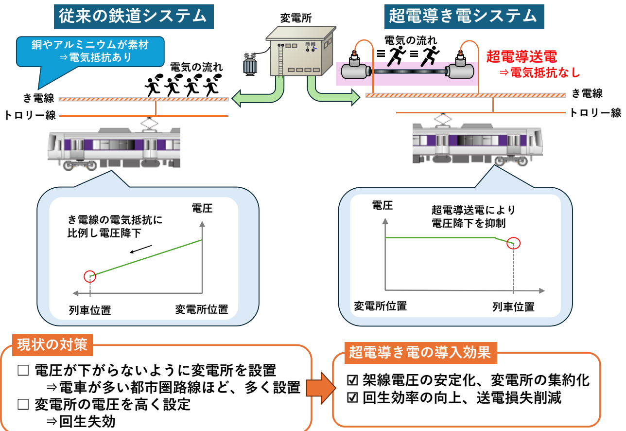
図2 超電導き電システムの概要
