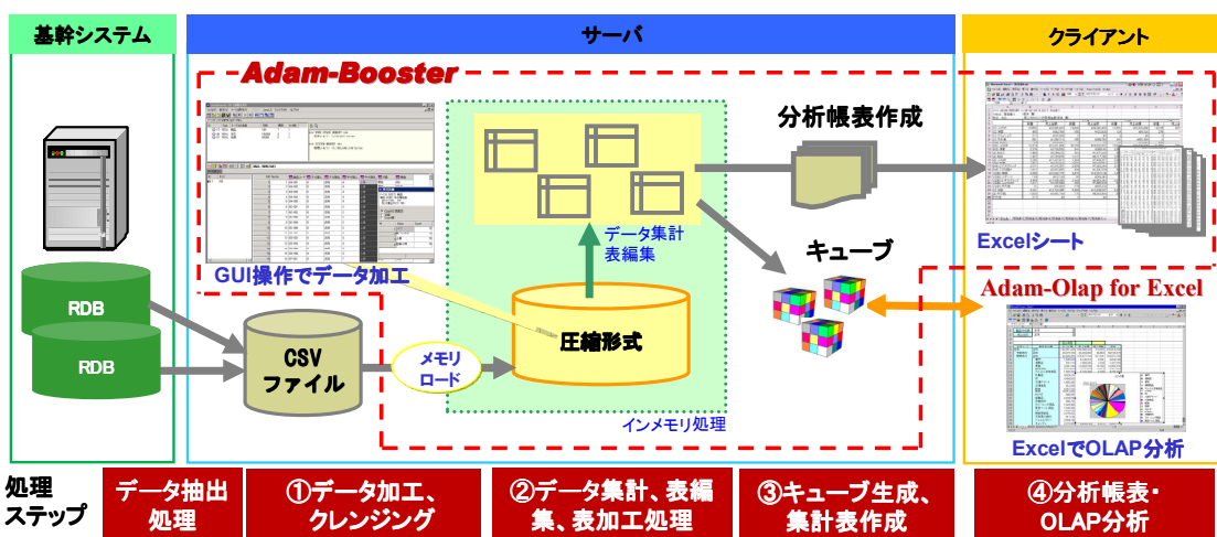
<Adam-Booster の全体概要>
