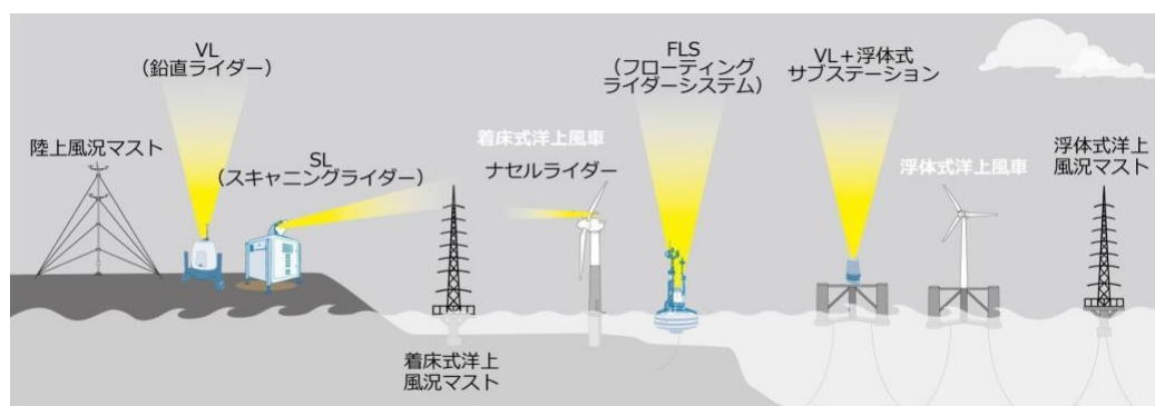
図4 風況観測機器の概略図（本試験サイトにない機器も図の中にも含まれます）
