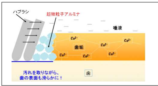
新採用の清掃剤アルミナによる清掃の仕組み
