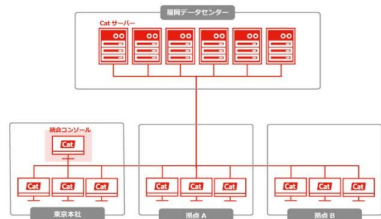
○SSJC ネットワーク構成図
